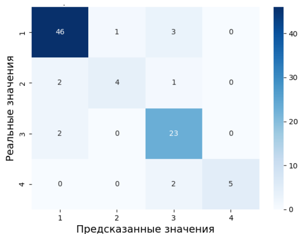
Рис. 3. Матрица ошибок модели LGBMClassifier (данная модель показала наилучшие результаты и точность в способности к рекомендациям).
